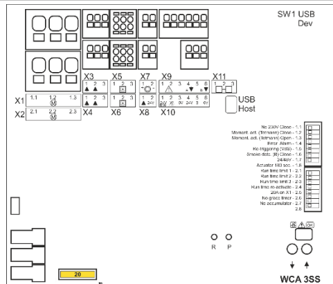
Placering af 20A flink sikring
